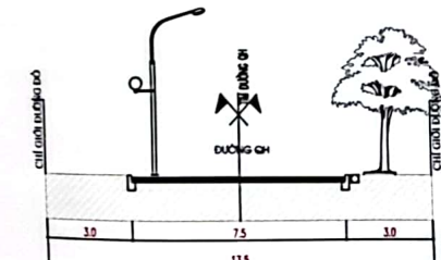
MẶT CẮT 2 - 2
