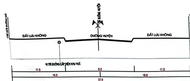
MẶT CẮT 1 - 1
